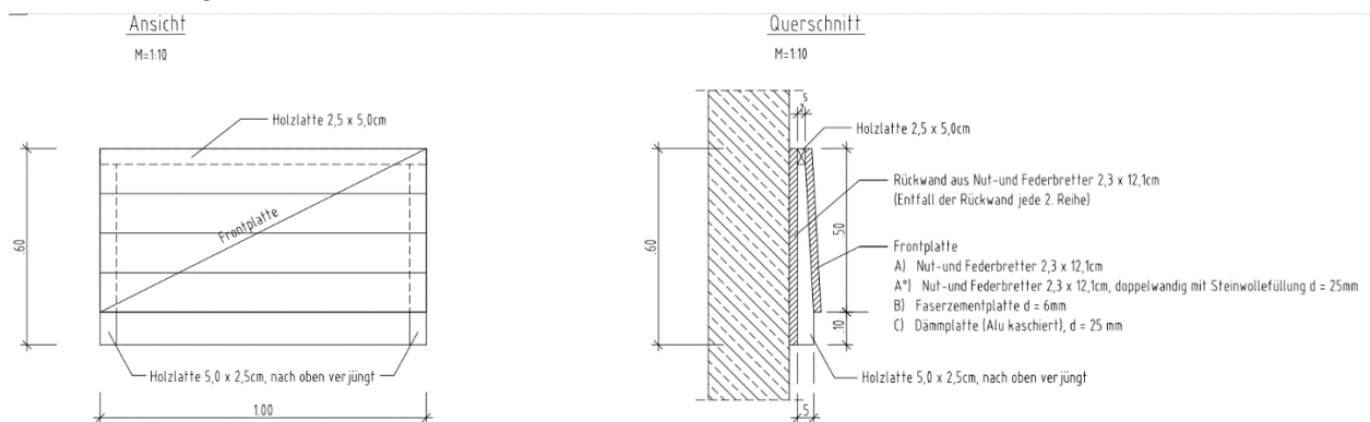
Abbildung 38: Detailzeichnung Fledermauslangkasten gemäß Maßnahme A6 CEF
